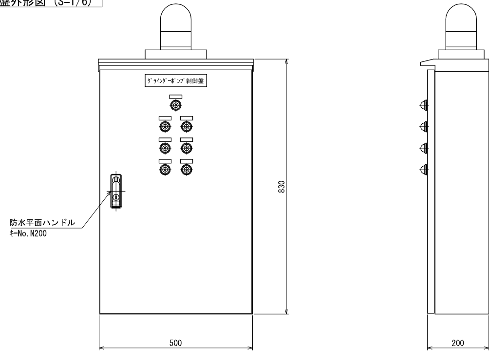
制御盤外形図 (S=1/6)
