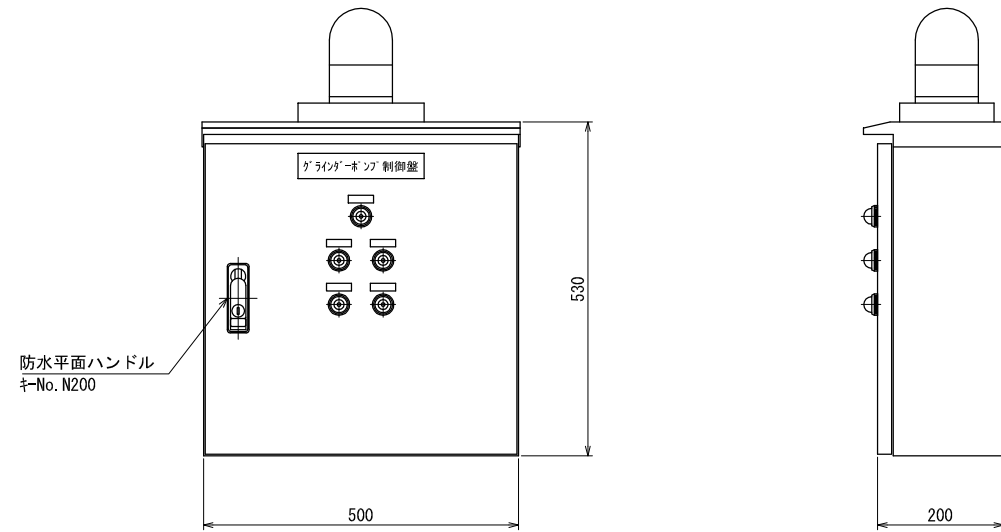
制御盤外形図 (S=1/6)
