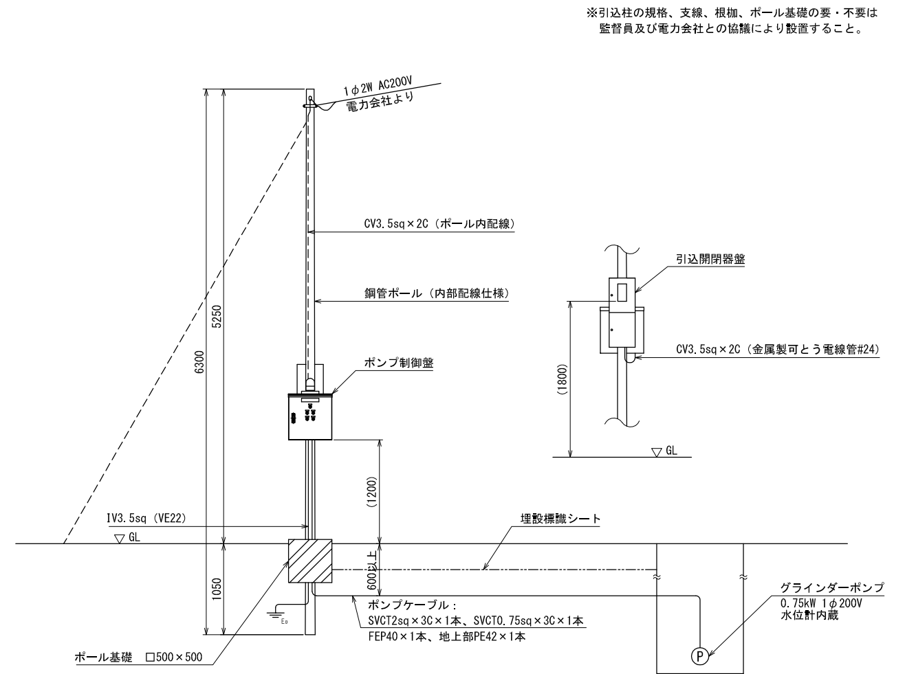
電気工事図 (S=1/30)
